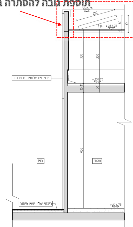
חתך עקרוני קולטן שמש במסגרת היתר שינויים
