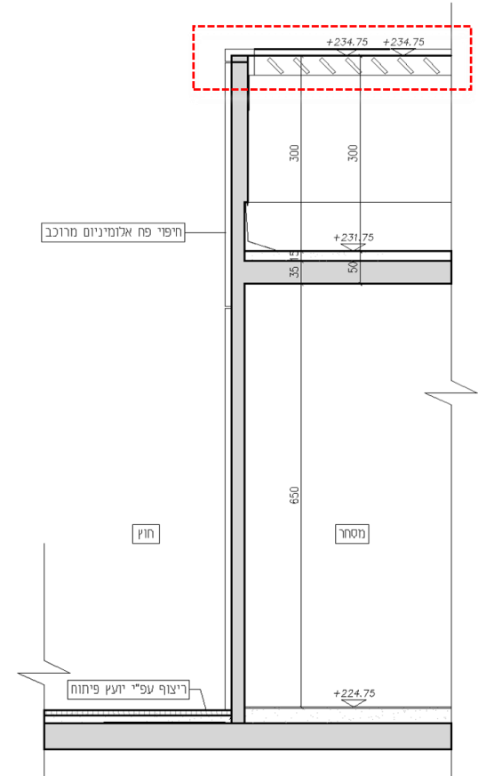
חתך עקרוני קירוי גג
